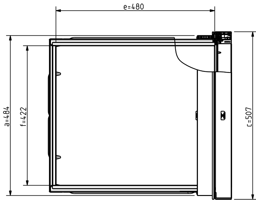
SEZIONE C-C
