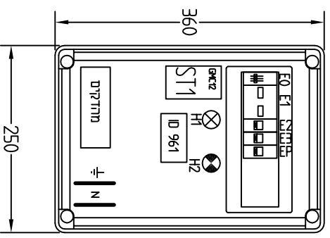
מבנה לודו קופסת C-4 עם קולפא
