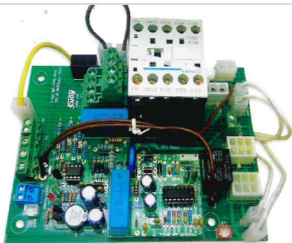
כרטיס מעבה למזגני אלקטרה/אלקו טייפון תלת פאזי מק"ט: USP-2003
