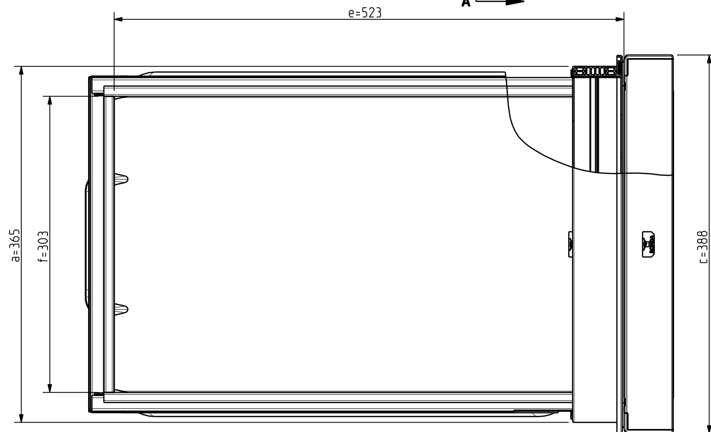
SEZIONE C-C
