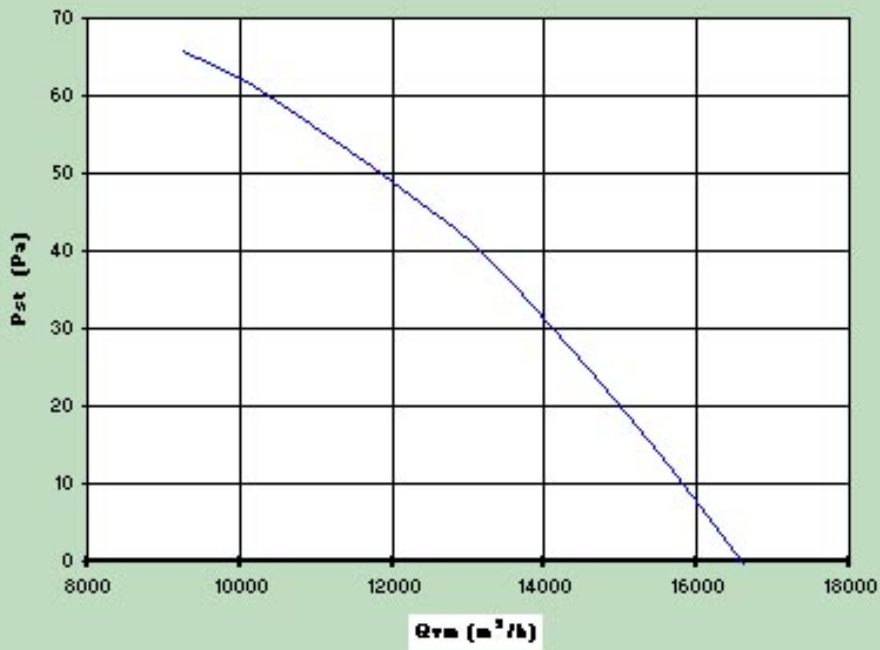
P=f(Qvm)
