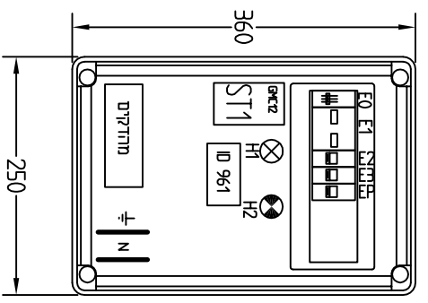
מבנה לוח קופסה C-4 עם קולפס
