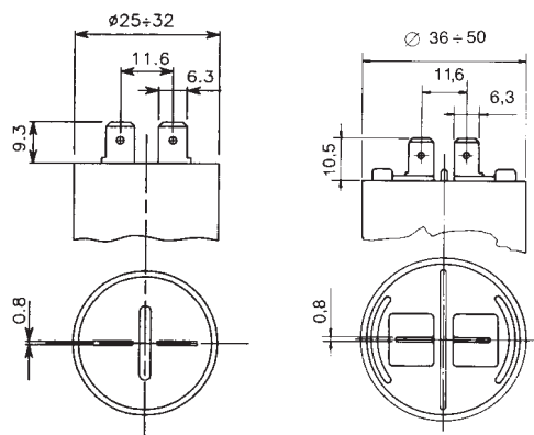
Fig. 2 Faston semplice 6,3 x 0,8 mm
