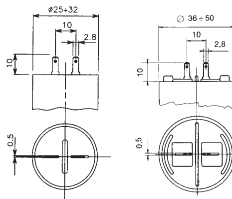
Fig. 3 Faston 2,8 x 0,5 mm
