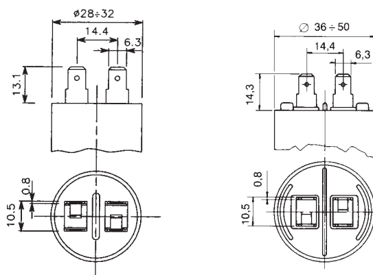
Fig. 1 Doppio Faston 6,35 x 0,8 mm
