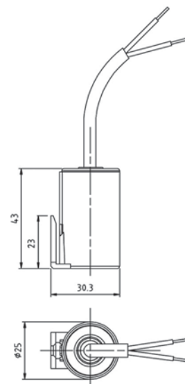
Fig. 8 Versione con fissaggio a linguetta solo in dim. Ø25x43
